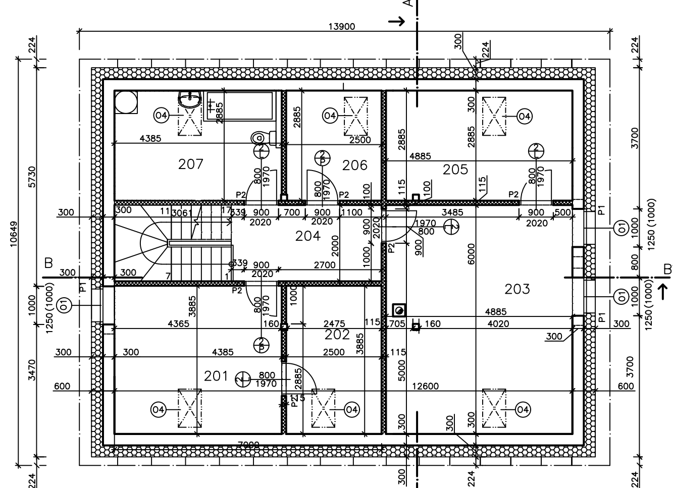
PŮDORYS 2.N.P.
