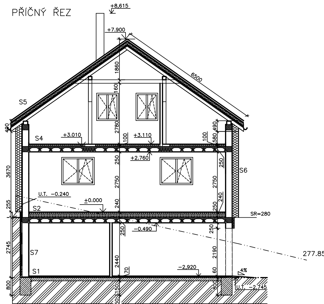
PRŮČNÝ ŘEZ
