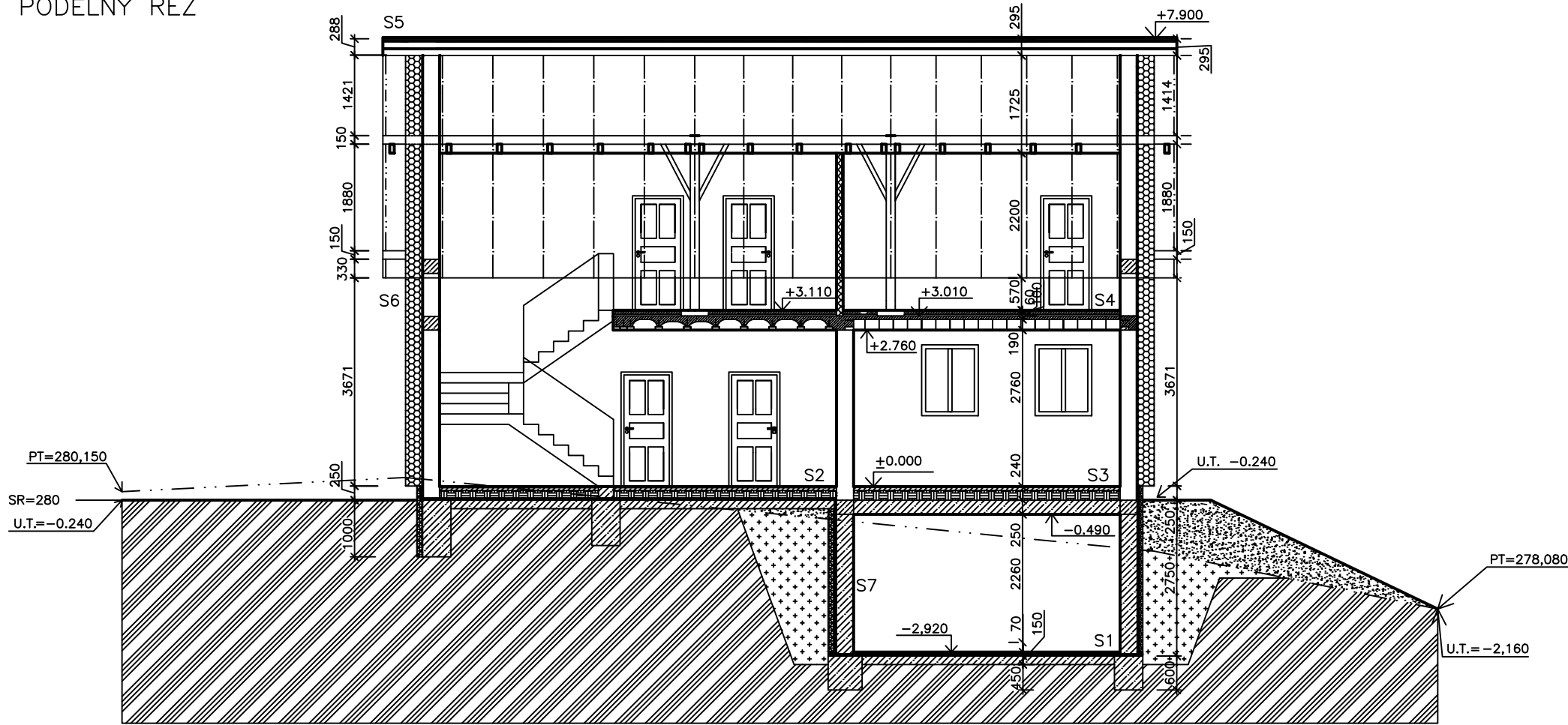
PODÉLNÝ ŘEZ
