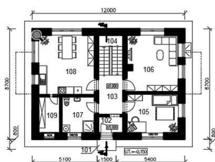
PÔDORYS 1. NP M 1:100
