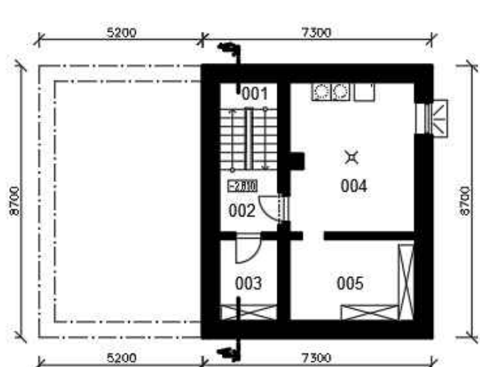
PÔDORYS 1. PP M 1:100
