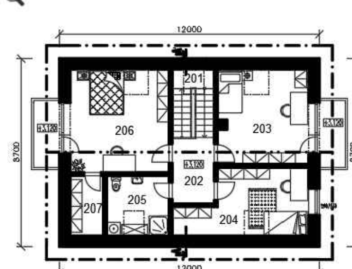
PÔDORYS 2. NP M 1:100
