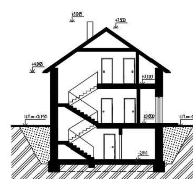
ZVISLÝ REZ A-A' M 1:100
