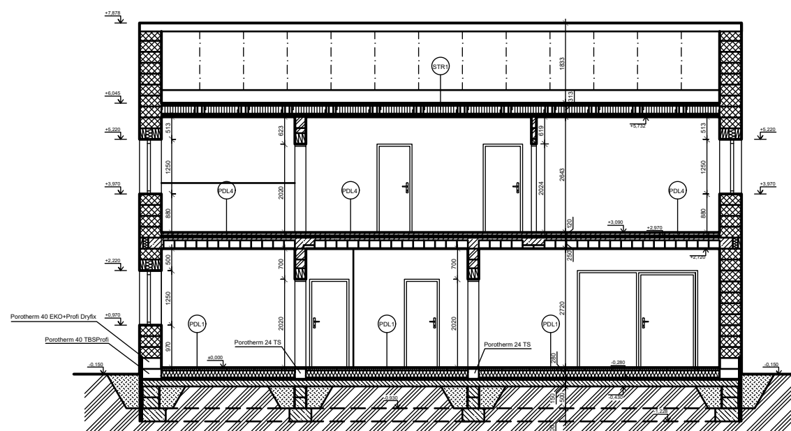
ŘEZ A-A'
