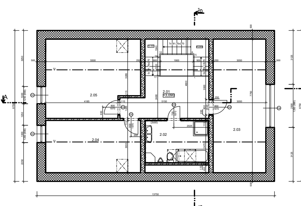
PŮDORYS 2.NP
