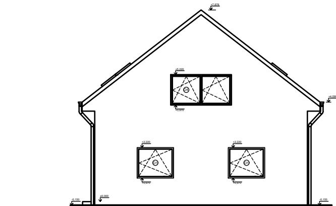
POHLED SEVEROVÝCHOD
