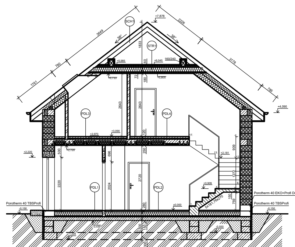
ŘEZ B-B'
