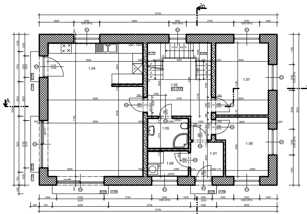
PŮDORYS 1.NP
