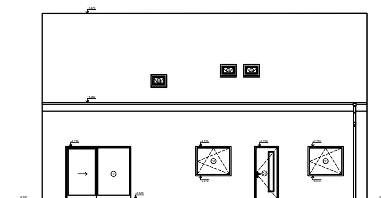
POHLED JIHOZÁPAD
