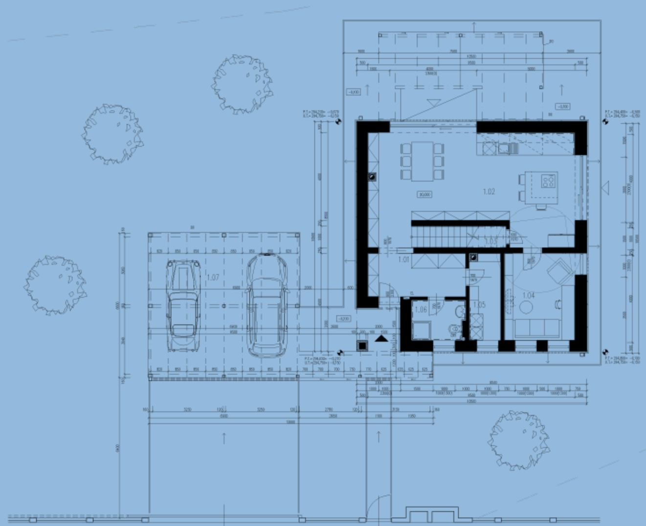
PŮDORYS 1.NP
