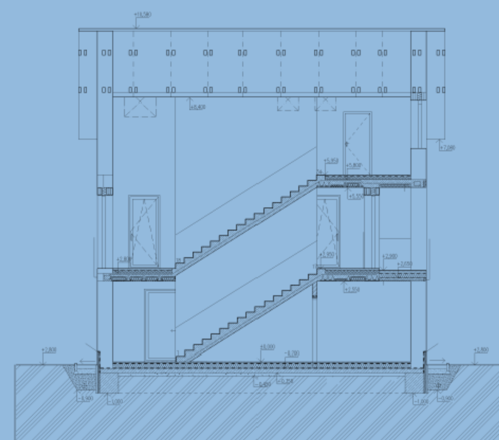
ŘEZ PŘÍČNÝ
