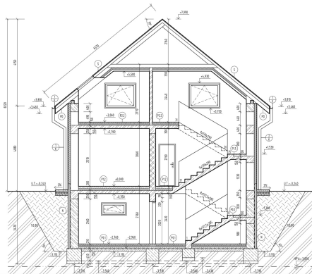
Rez A-A'
