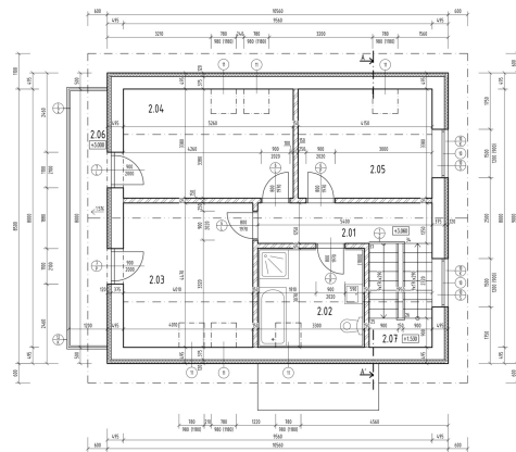
Pôdorys 2.NP
