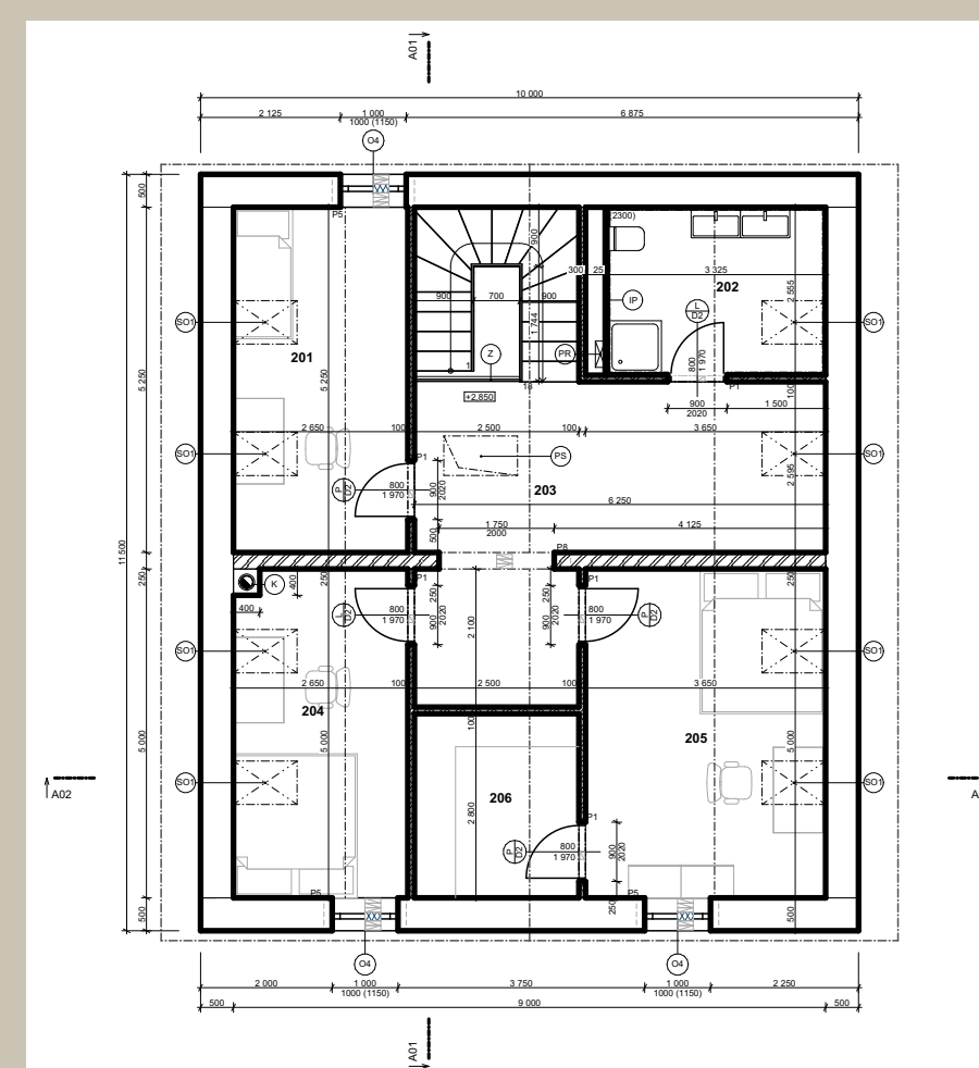
PŮDORYS PODKROVÍ
