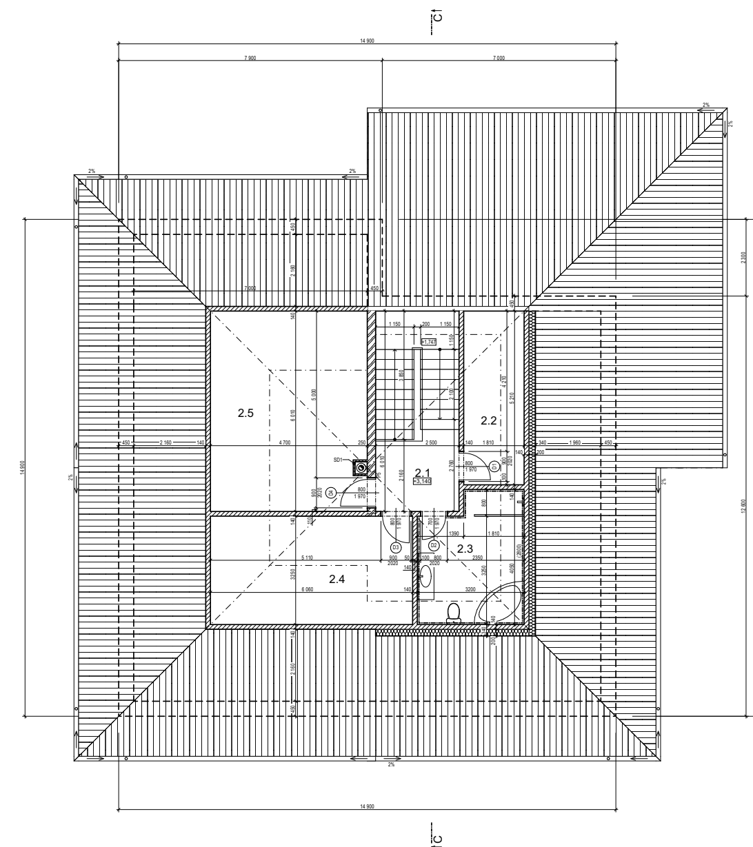
PŮDORYS 2.NP
