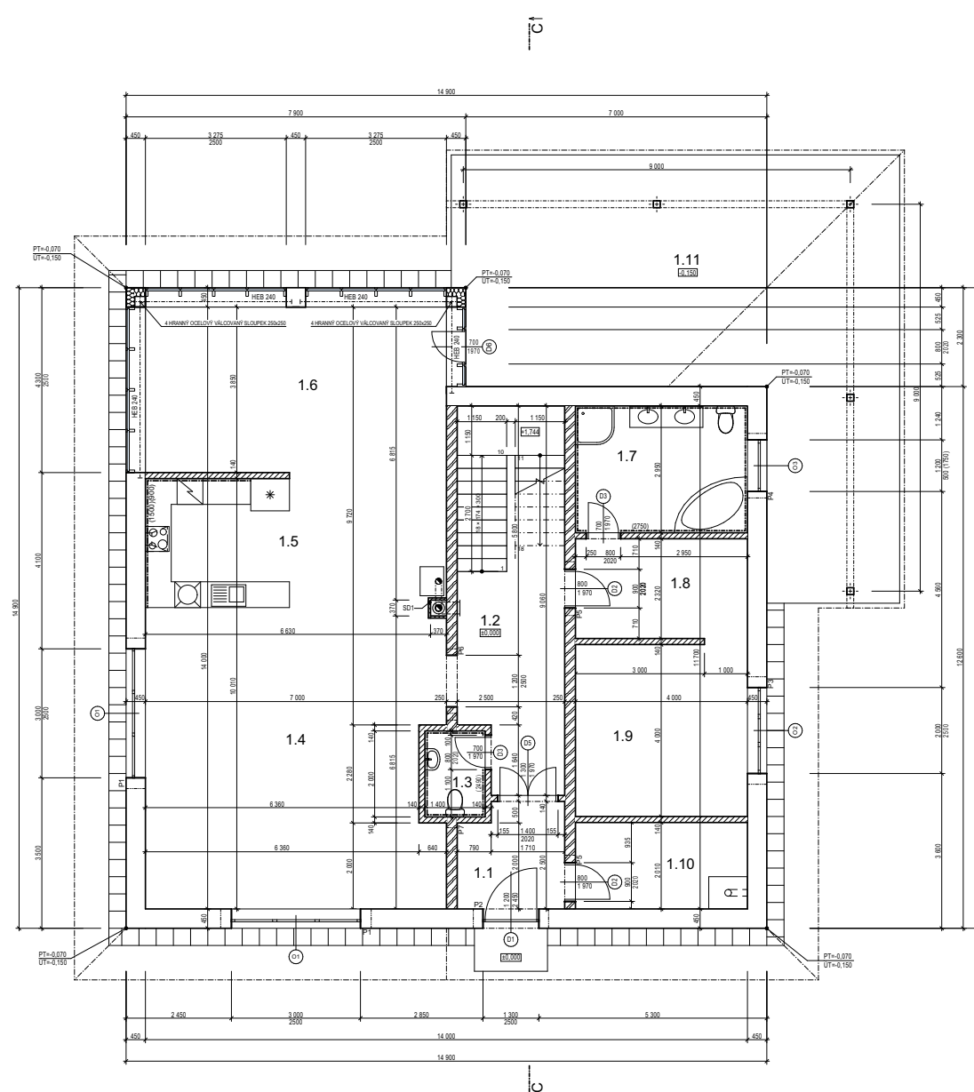
PŮDORYS 1.NP
