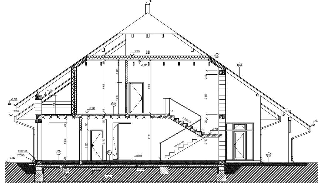
ŘEZ
