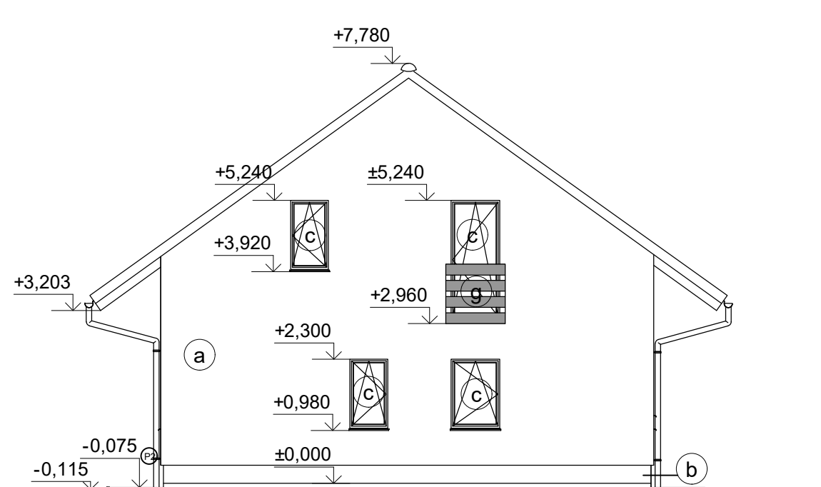
POHLAD VÝCHODNÝ
