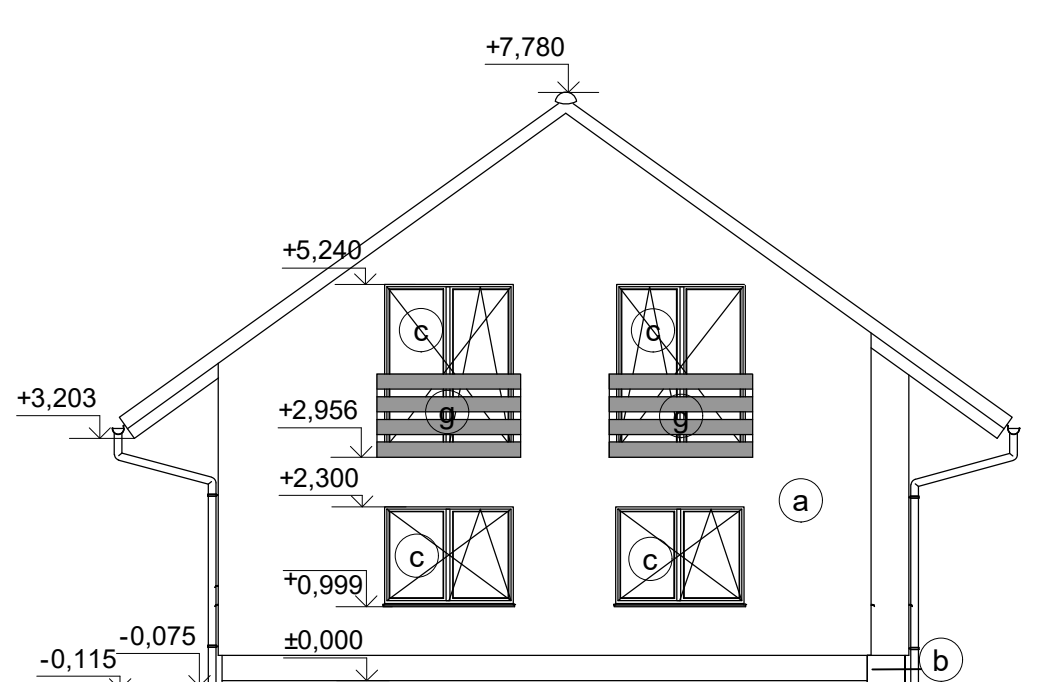
POHLAD ZÁPADNÝ
