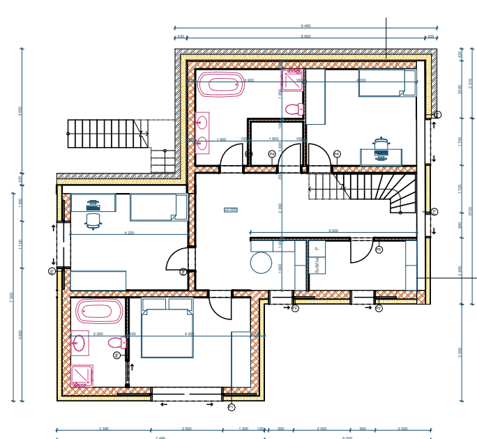
Půdorys 1.NP
