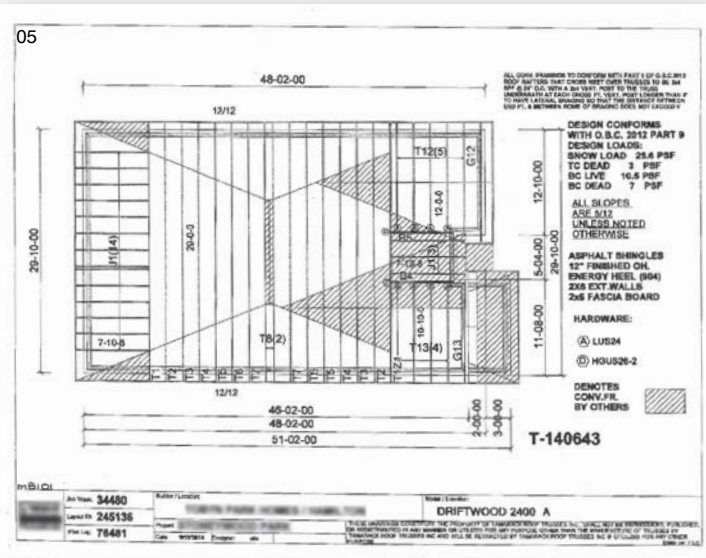
05) Ukázka dílenských výkresů základy
